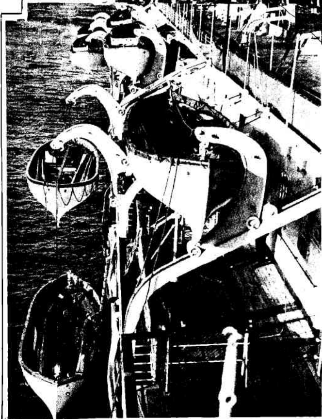
LA CATASTROFE DEL "VESTRIS" ha hecho que los constructores de buques piensen en perfeccionar el sistema de lanzamiento de los botes salvavidas. He aquí un nuevo procedimiento que permite lanzar al agua 6 botes en un minuto. Este sistema ha sido instalado en el "Duquesa de Bedford", de la Canadian Pacific Line.
