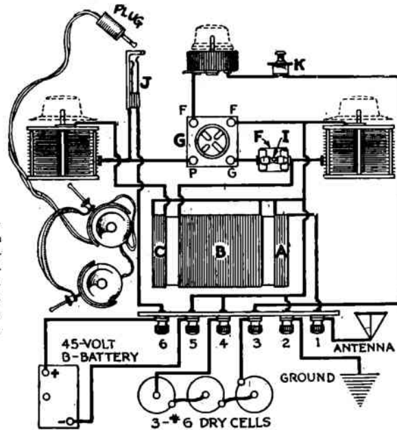
Fig. 2 Diagrama explicativo de la forma en que van conectadas entre sí, las piezas del equipo incluyendo la antena, tierra, baterías "A" y "B" y los teléfonos.
